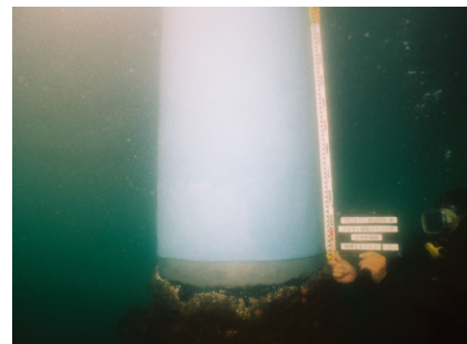
鋼管杭被覆状況(水中)
