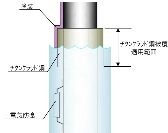
干満帯近傍の防食仕様例
